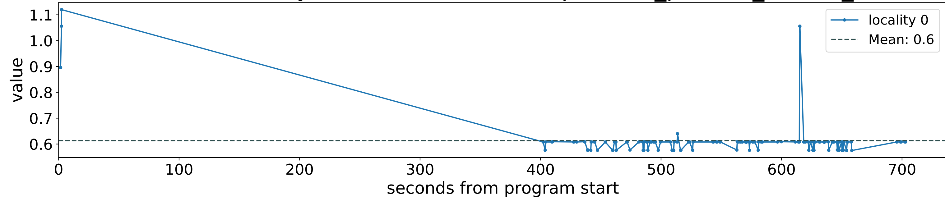
GPU: submit delay (us): void Kokkos::Impl::cuda_parallel_launch_loc...
