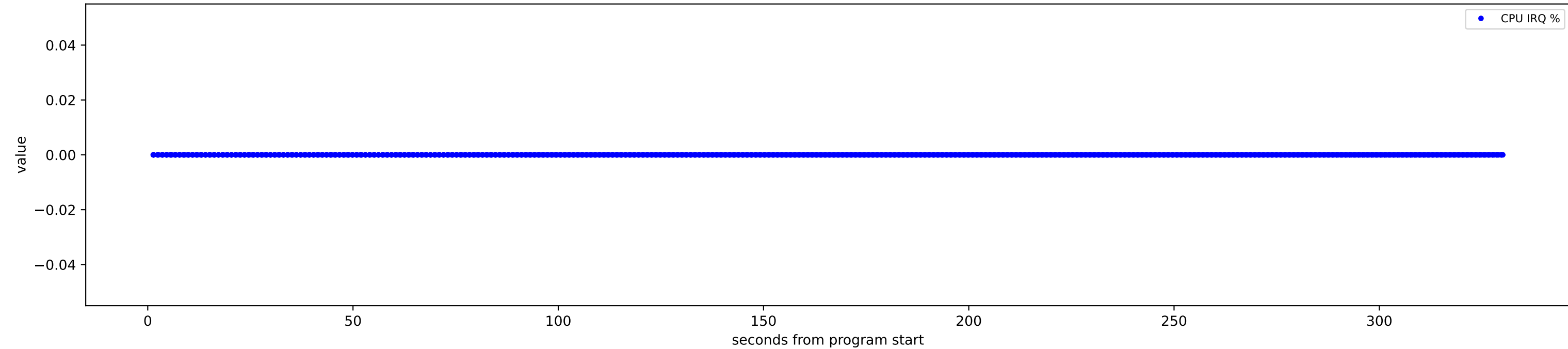
CPU IRQ %
